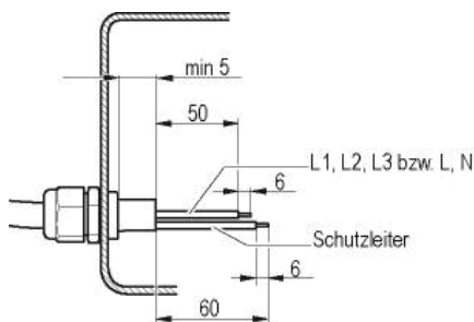
Abb. 1: Empfohlene Abmantellungsgrößen in mm (innerhalb Klemmkasten)
